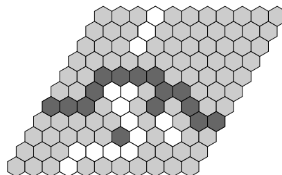
FIGURE 1 – Une partie de Hex sur un plateau 11 \times 11 .
