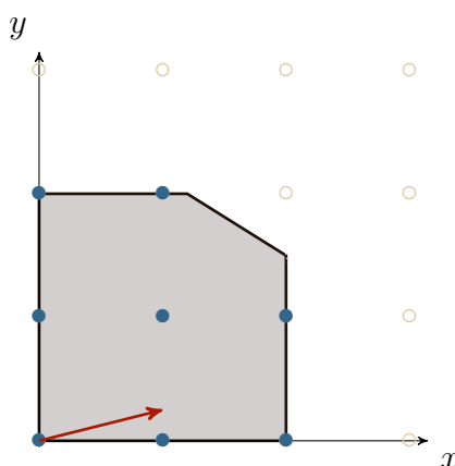
(a) Une instance de OLNE
