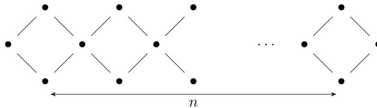
FIGURE 4 – Graphe G_n sur lequel l'algorithme GloutonStable est mauvais
