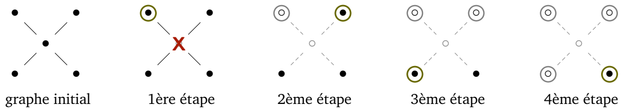
FIGURE 2 – Exécution de StableGlouton conduisant à une solution optimale
