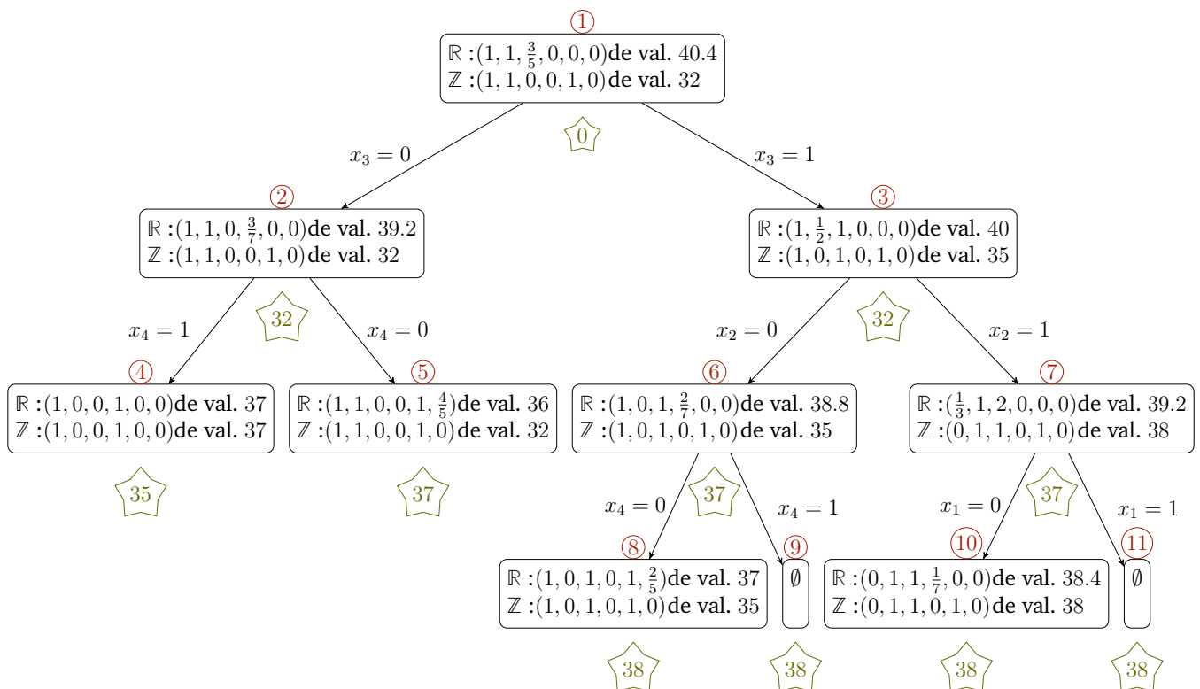
FIGURE 9 – Exécution de l'algorithme 6 sur l'instance exemple
