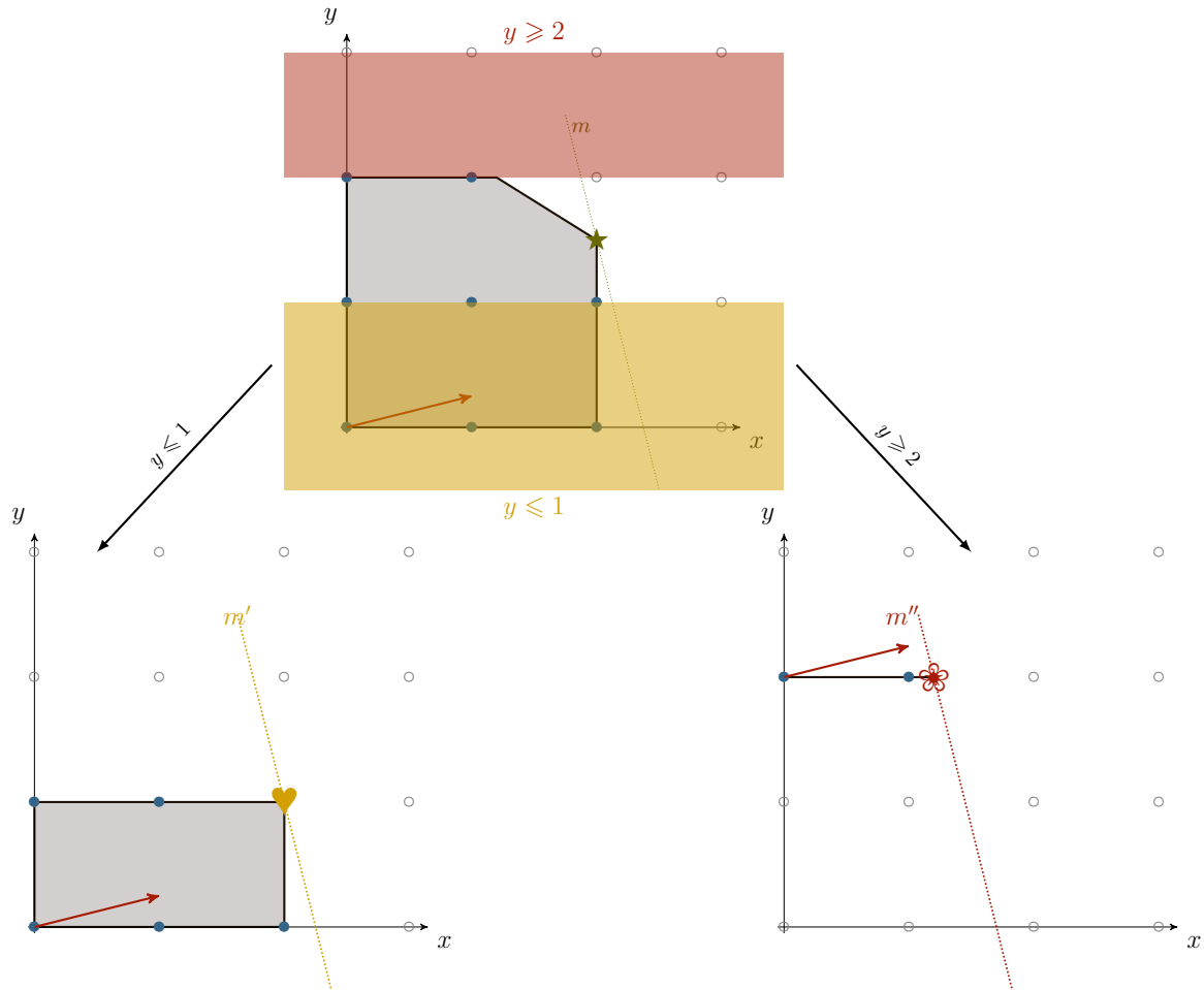
FIGURE 8 – Une étape de découpage
