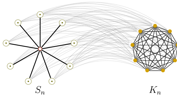
FIGURE 5 – Graphe G'_n sur lequel l'algorithme GloutonStable est très mauvais
