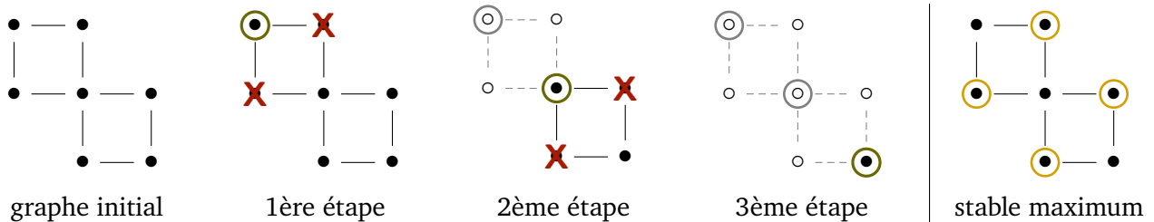
FIGURE 3 – Exécution de StableGlouton conduisant à une solution approchée (de rapport \frac{3}{4} = 0.75 )
