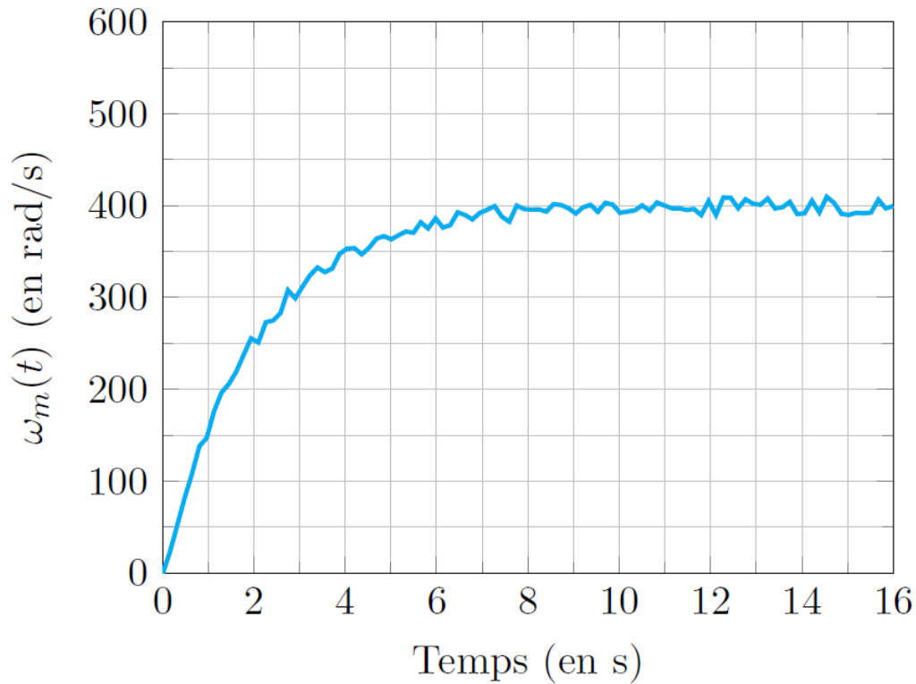
FIGURE 8 – Réponse indicielle du moteur
