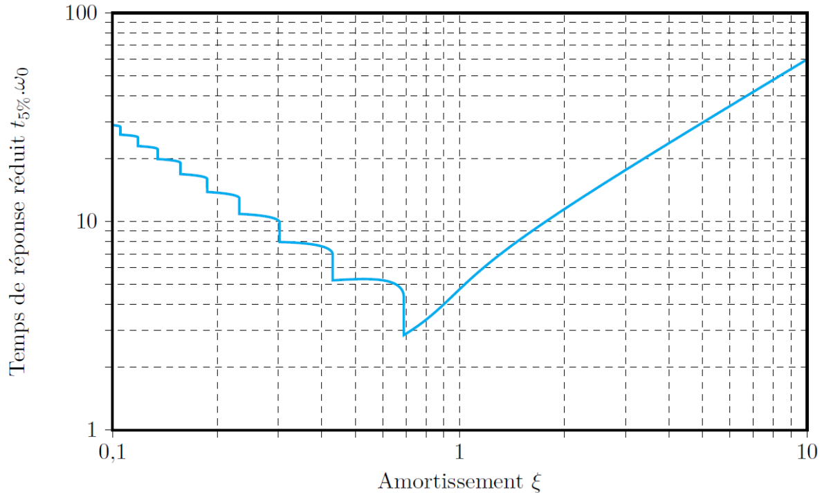
FIGURE 9 – Abaque des temps de réponse réduits d'un système d'ordre 2 de classe nulle
