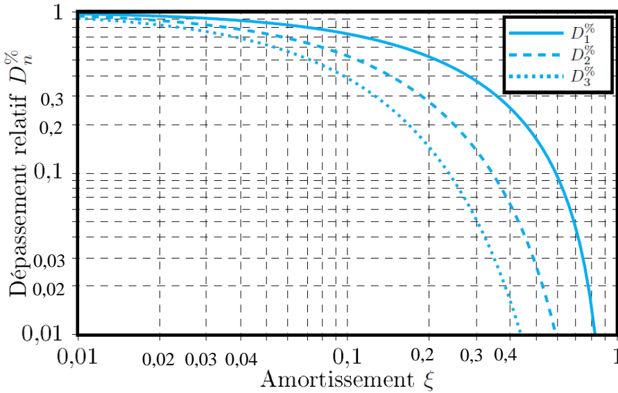
Figures 15 : Abaqués à échelles logarithmiques des dépassements relatifs et du temps de réponse réduit pour un système du 2 ème ordre
