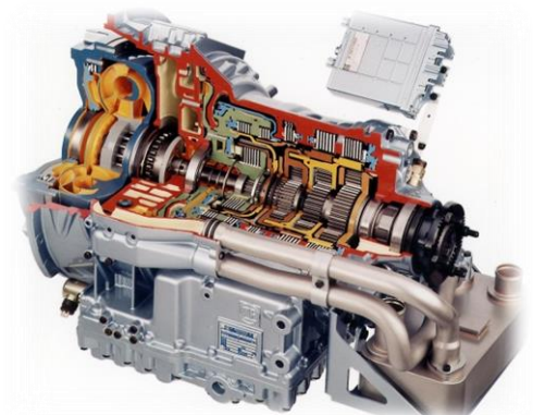
Boîte de vitesses automatique à 3 trains épicycloïdaux
