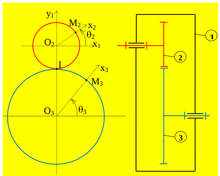
schéma cinématique : représentation symbolique normalisée à connaître
