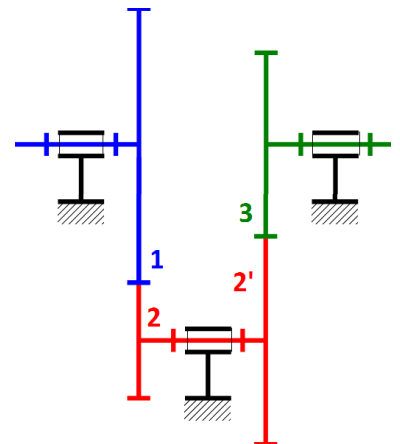
Schéma cinématique
