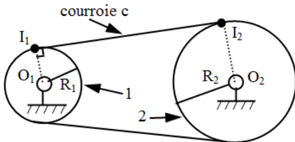
Schéma cinématique système poulie courroie
