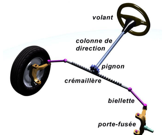
Crémaillère de direction de voiture
