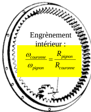
Engrenages à denture intérieure
