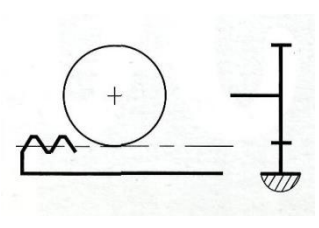
Pignon crémaillère photo et schéma cinématique
