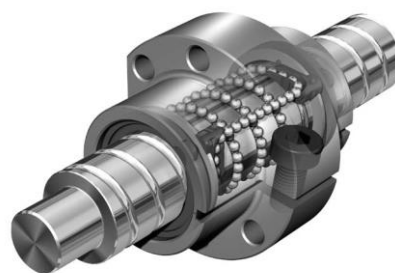
Vis/écrou à billes (bras maxpid)
