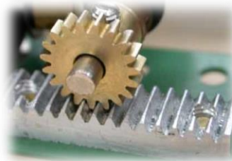
Pignon crémaillère photo et schéma cinématique
