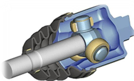
joint tripode (celui des voitures)
