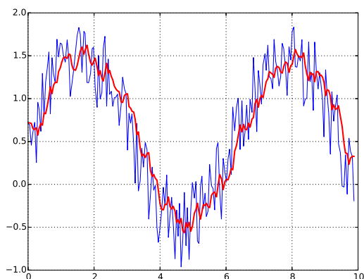
FIGURE 2 – Débruitage par filtre passe-bas RC pour différentes valeurs de \tau
