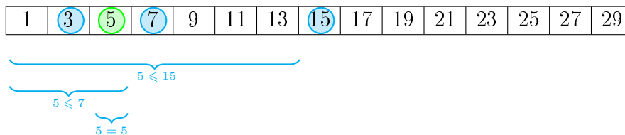
FIGURE 1 – Recherche dichotomique de 5 dans [1, 3, \dots, 29]
