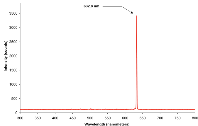
FIGURE 6 – Spectre d'un LASER He-Ne (hélium-néon)
