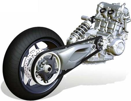
Transmission par courroie crantée
