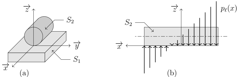
FIGURE 7 – Paramétrage du contact cylindre-plan (a) et action mécanique linéique (b).
