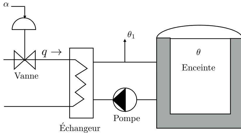
FIGURE 5.1 – Enceinte chauffée.
