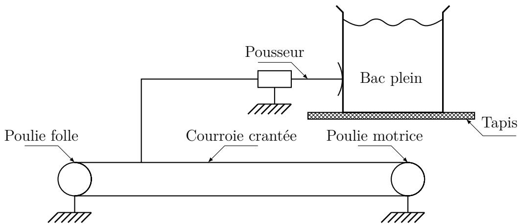
FIGURE 3.1 – Shématisation d'un modèle d'éjection.
