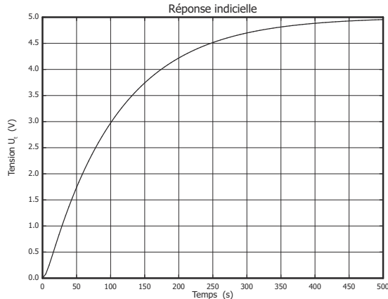
FIGURE 7.3 – Réponse indicielle du système.
