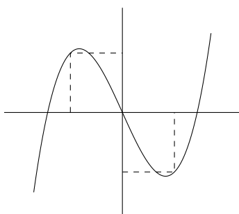
fonction impaire
