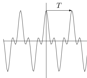
fonction périodique
