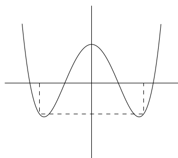
fonction paire
