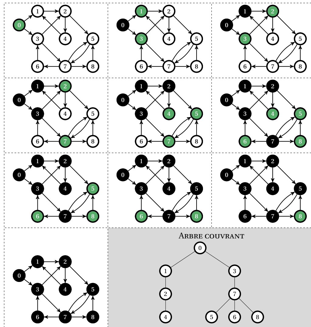
Figure 6 – PARCOURS EN LARGEUR D'UN GRAPHE ORIENTÉ
