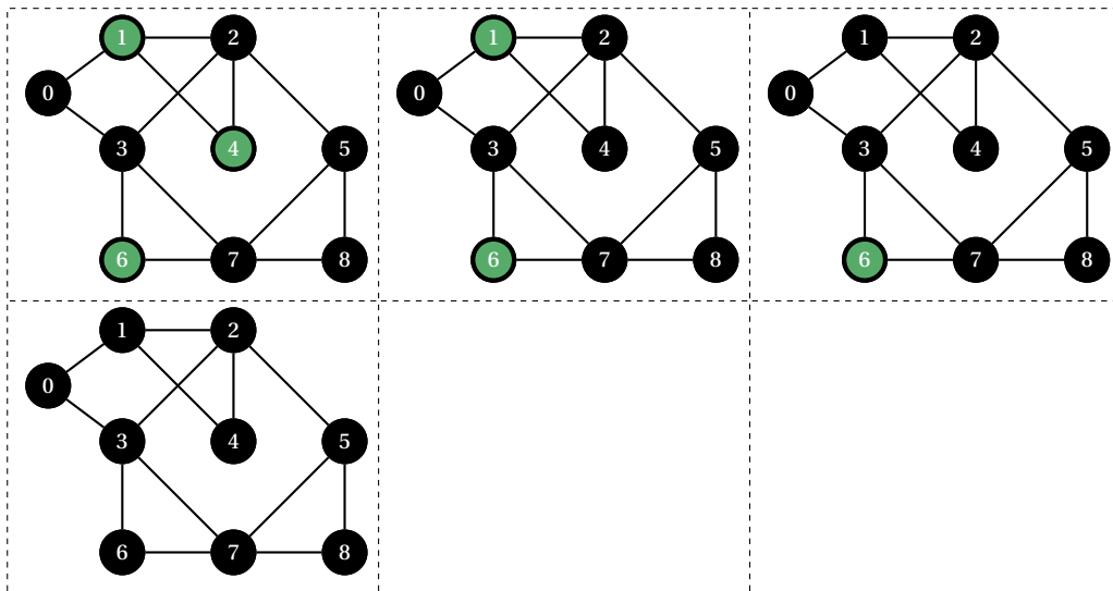
PARCOURS EN PROFONDEUR D'UN GRAPHE NON ORIENTÉ.
