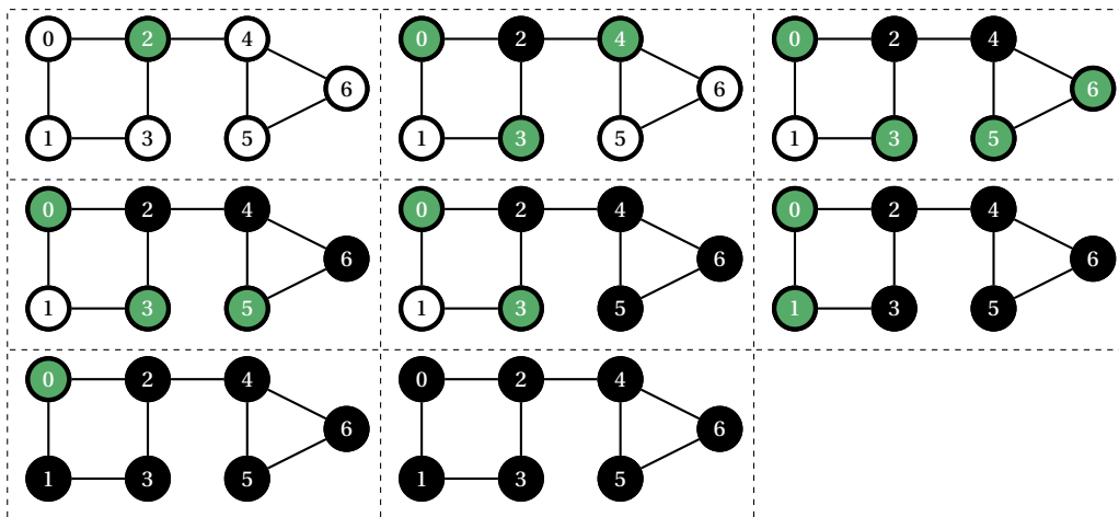
Figure 3 – PARCOURS EN PROFONDEUR D'UN GRAPHE NON ORIENTÉ.
