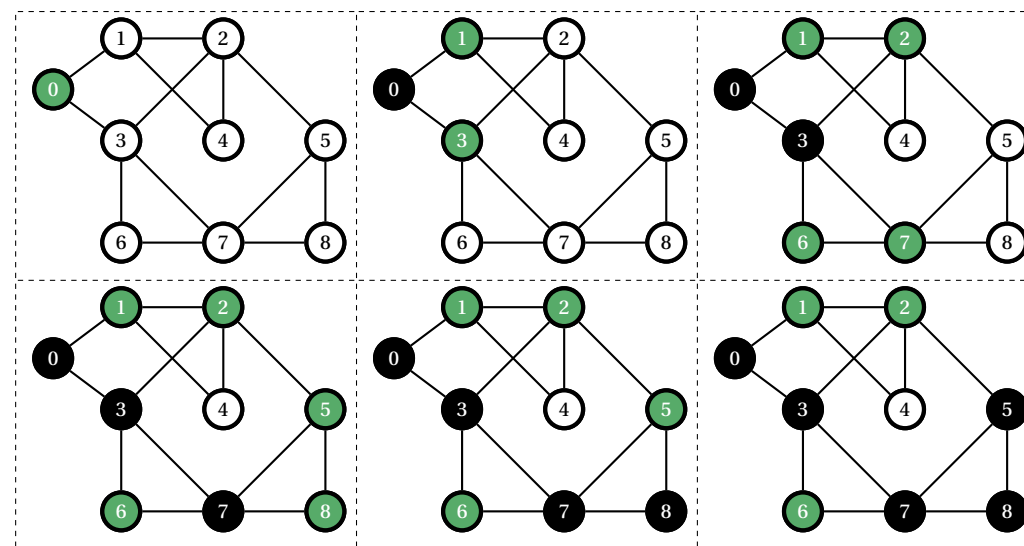
Figure 2 – PARCOURS EN PROFONDEUR D'UN GRAPHE NON ORIENTÉ.
