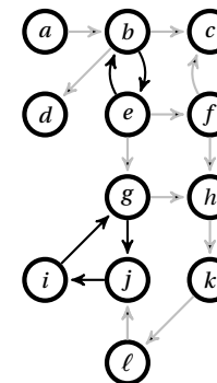
FIGURE 14. – Deux cycles dans un graphe orienté.
