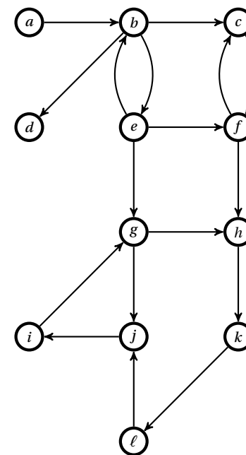
FIGURE 11. – Graphe orienté et chemins.
