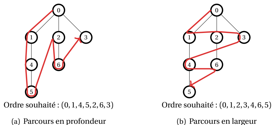
FIGURE 1. – Deux types de parcours
