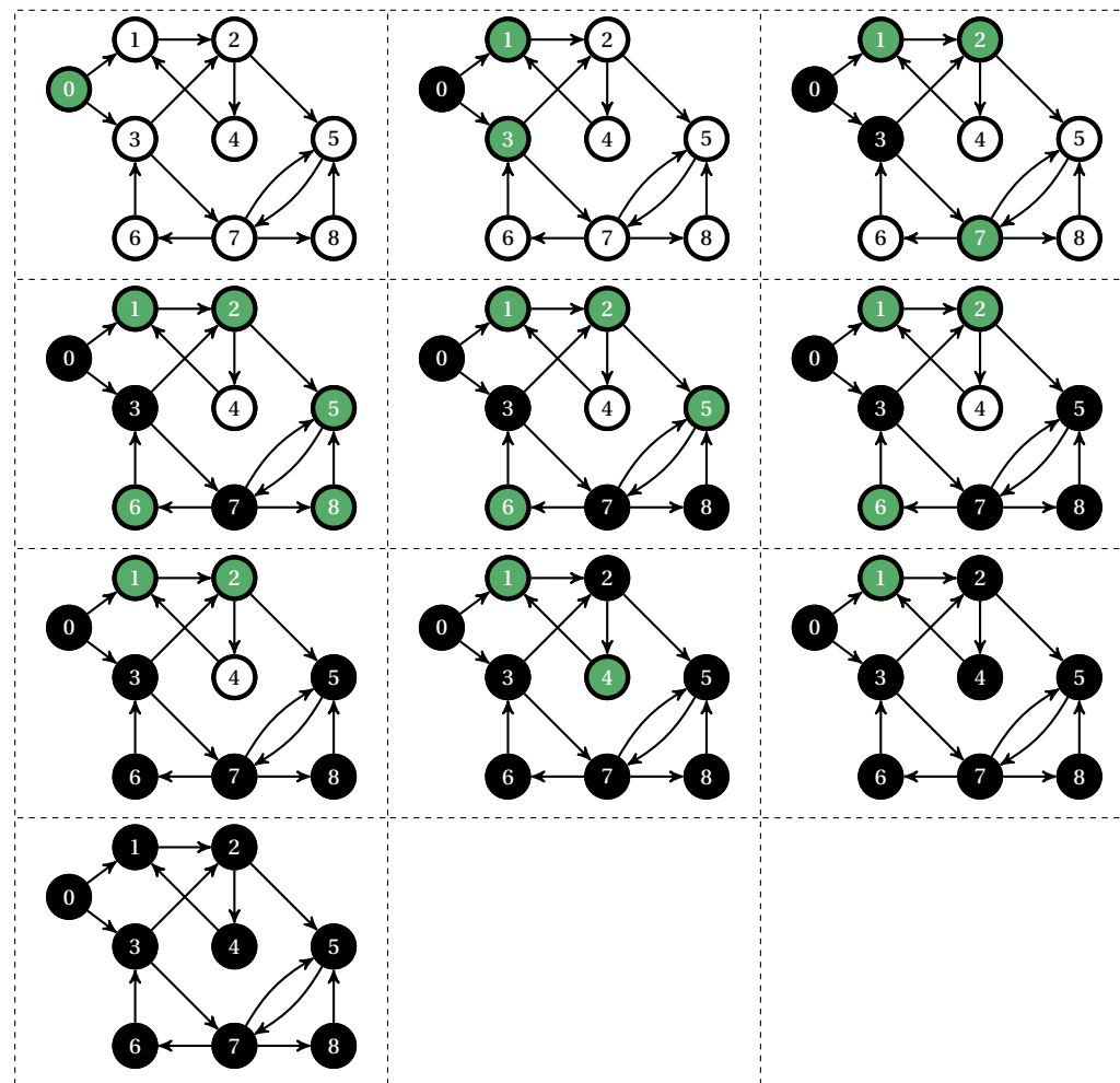
Figure 4 – PARCOURS EN PROFONDEUR D'UN GRAPHE ORIENTÉ.
