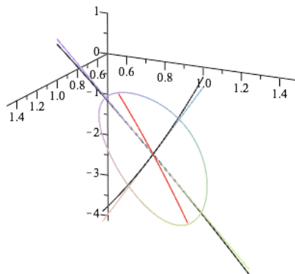
REPRÉSENTATION DU GRADIENT EN ROUGE, DIRECTION DE L'ACCROISSEMENT MAXIMALE DE f
