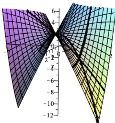
LIGNES DE REPRÉSENTATION DE \varphi_{\vec{u}} ET DÉRIVÉES PARTIELLES
