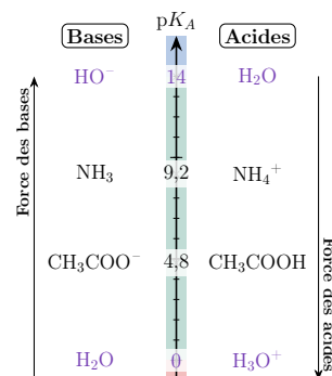
FIGURE TM4.4 – Échelle \text{p}K_A
