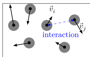
Gaz Réel
