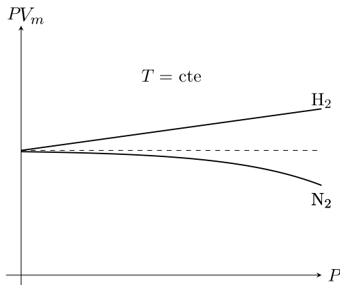
FIGURE T1.3 – Diagramme d'AMAGAT pour deux gaz distincts à faible pressions.
