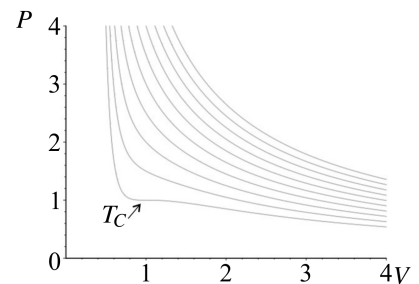
FIGURE T1.5 – Isothermes réelles en (P, v) .
