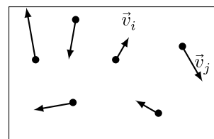
Modèle du gaz parfait
