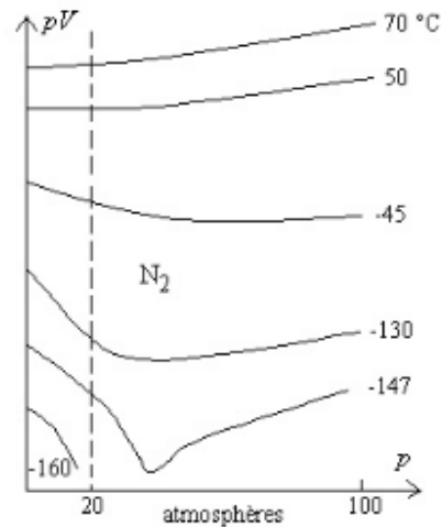
FIGURE T1.4 – Diagramme d'AMAGAT pour le diazote à différentes températures.
