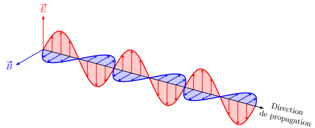
FIGURE O1.1 – Représentation des oscillations du champ électromagnétique lors de la propagation de la lumière
