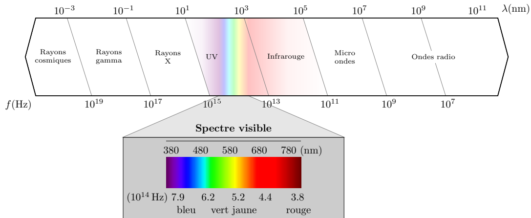
FIGURE O1.2 – Longueurs d'ondes des ondes monochromatiques dans le vide.
