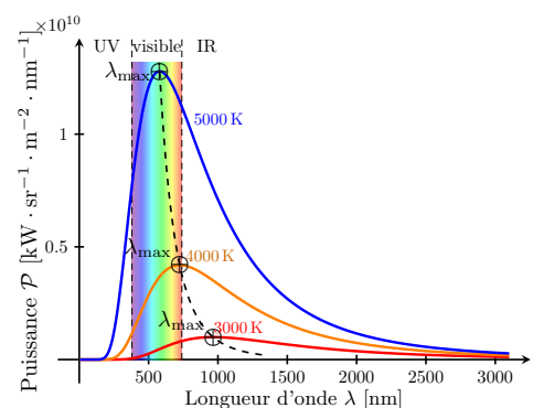
FIGURE O1.4 – Spectre d'émission d'un corps chaud.
