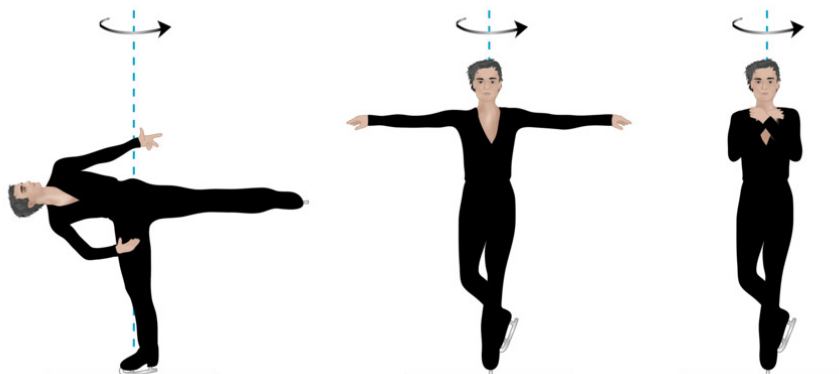
FIGURE M8.5 – Un-e patineur-euse accélère en rapprochant ses bras de son corps
