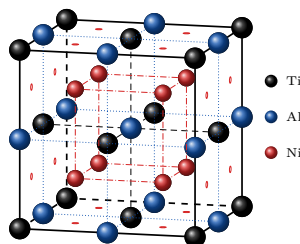
FIGURE AM5.2 – Maille élémentaire de l'alliage. Les couleurs sont indiquées dans la légende.
