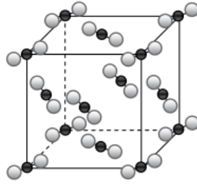
FIGURE AM5.3 – Maille élémentaire de carboglace. Le carbone est en noir, l'oxygène en gris.
