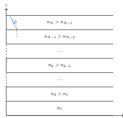
FIGURE O2.3 – Modèle d'atmosphère stratifiée
