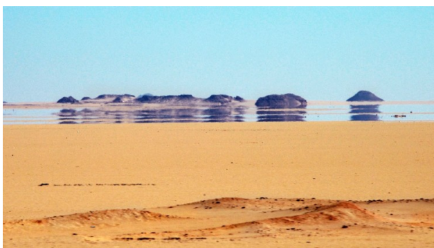
FIGURE O2.2 – Photo d'un mirage chaud
