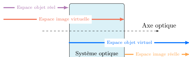
FIGURE O2.17 – Espaces objet et image.
