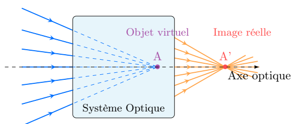
FIGURE O2.15 – Objet virtuel et image réelle.
