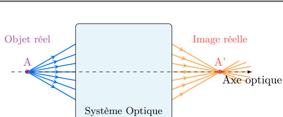
FIGURE O2.13 – Objet et image réelles.
