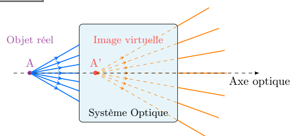
FIGURE O2.14 – Objet réel et image virtuelle.
