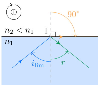
Réfraction limite : i_1 = i_{\text{lim}}
