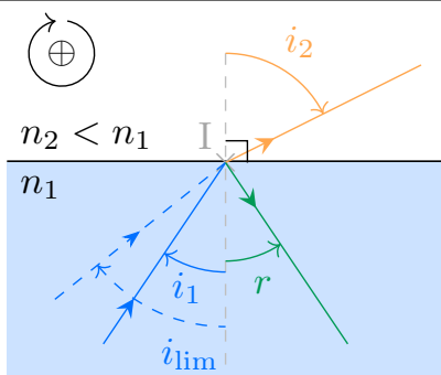
Réfraction : i_1 < i_{\text{lim}}
