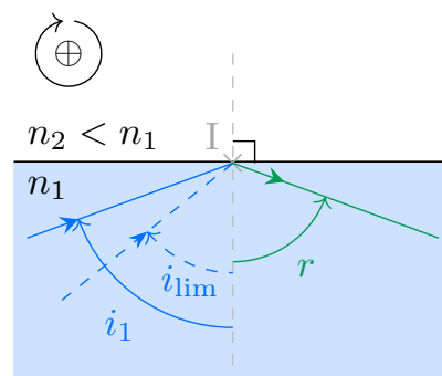
Réflexion totale : i_1 > i_{\text{lim}}
