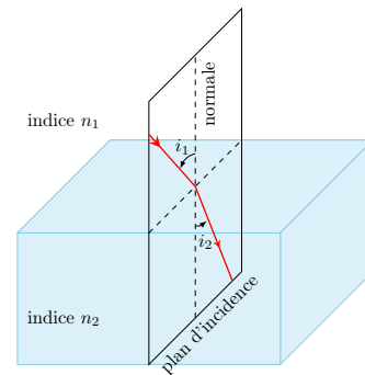
FIGURE O2.7 – Réfraction.
