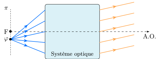
FIGURE O2.21 – Foyer secondaire objet.
