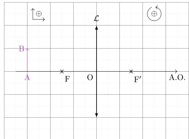
FIGURE O3.8 – Utilisation des règles principales
