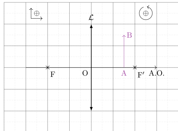
FIGURE O3.10 – Convergente après
