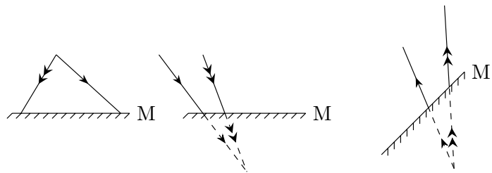
FIGURE O3.1 – Constructions optiques de miroirs plans.
