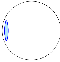
Œil myope au repos, obj. \infty
