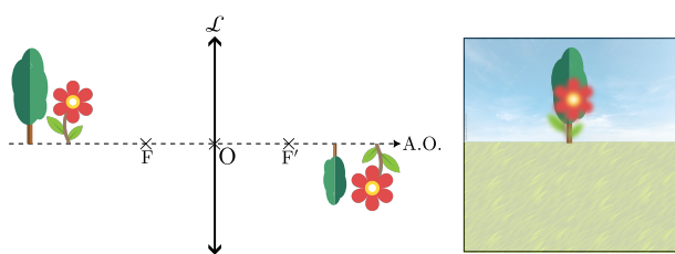
FIGURE 04.18 – Mise au point sur un arbre.
