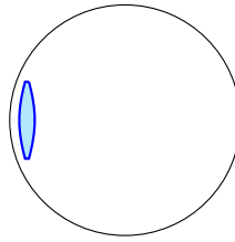
Œil hypermétrope au repos, obj. R
