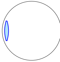
Œil hypermétrope au repos, obj. \infty
