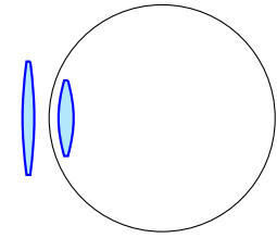
Œil hypermétrope au repos, corrigé
