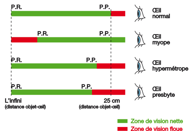
FIGURE O4.6 – Schéma des défauts de l'œil.
