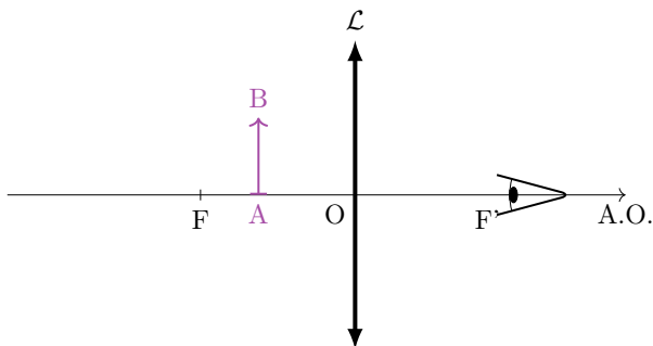
FIGURE O4.8 – Loupe avec accommodation
