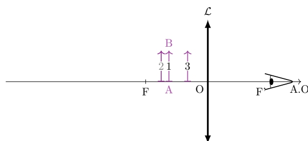
FIGURE O4.12 – Image obtenue avec une loupe dans plusieurs cas de distance objet-lentille
