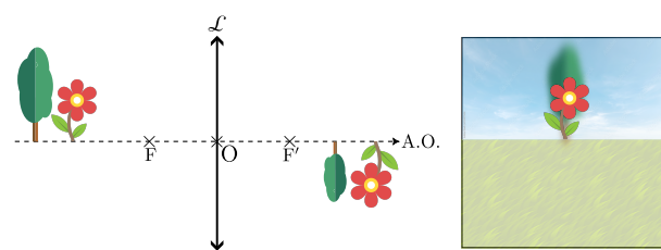
FIGURE 04.19 – Mise au point sur la fleur devant.
