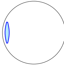
Œil myope au repos, obj. R
