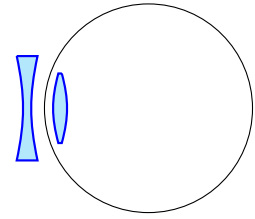
Œil myope au repos, corrigé
