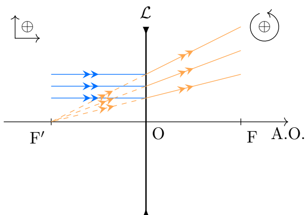
FIGURE O3.11 – e – Divergente faisceau parallèle
