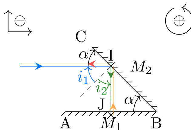
FIGURE O3.1 – Schéma du système
