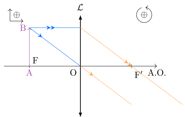
FIGURE O3.2 – b – Convergente sur F
