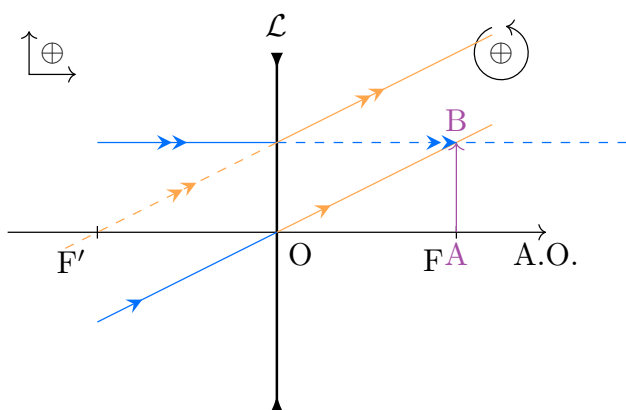
FIGURE O3.9 – c – Divergente sur F
