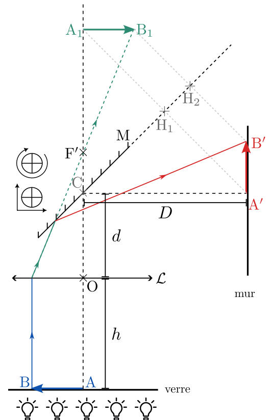
FIGURE O3.4 – Rétroprojecteur complété
