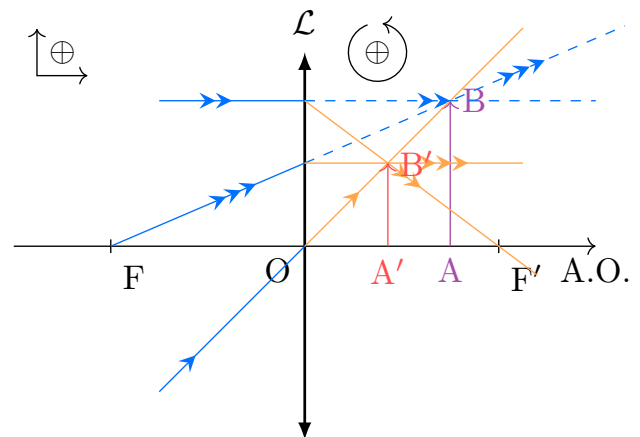
FIGURE O3.4 – d – Convergente après O
