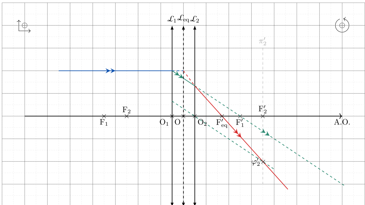
FIGURE TDO4.1 – Théorème des vergences pour deux lentilles accolées.
