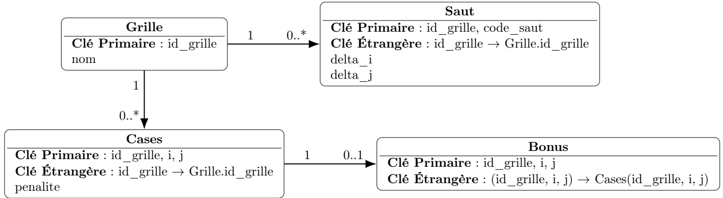
FIGURE 1 – Schéma relationnel avec clés primaires et étrangères
