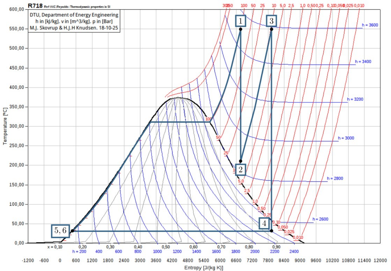
Figure 3 – Diagramme entropique complété.
