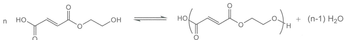
Figure 6 - Exemple de formation des polyesters insaturés (UP).
