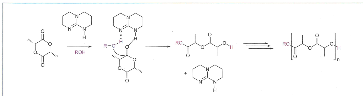
Figure 3 - Polymérisation du L-lactide via un mécanisme par liaison hydrogène à l'aide d'un organocatalyseur (ici la TBD) et d'un alcool en tant qu'amorceur.
