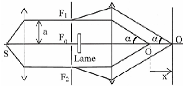
FIGURE 2 – Déplacement de l'écran
