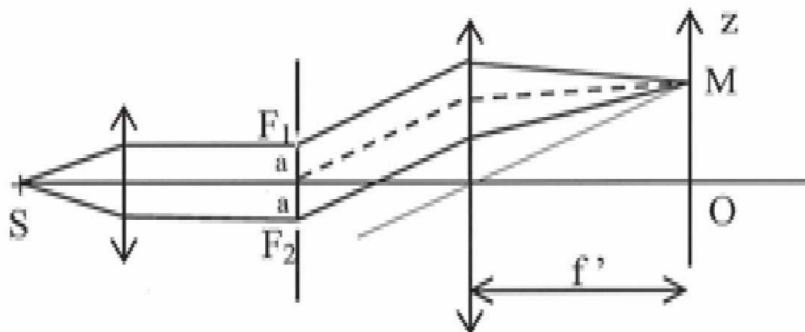
FIGURE 1 – Dispositif interférentiel à deux fentes
