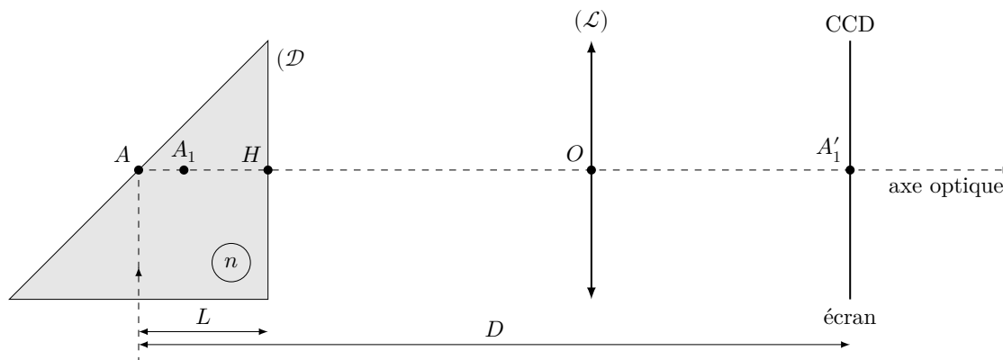
Figure 3 Schéma optique
