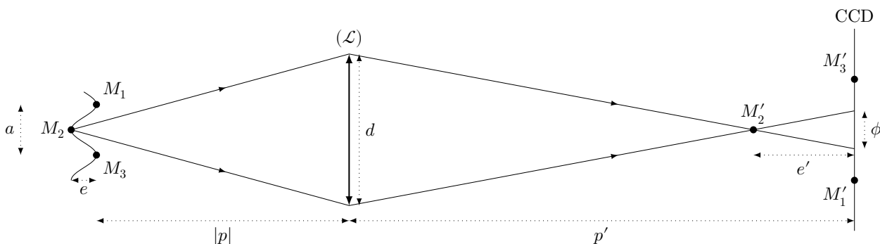
Figure 6 Formation de l'image d'un sillon d'empreinte digitale
