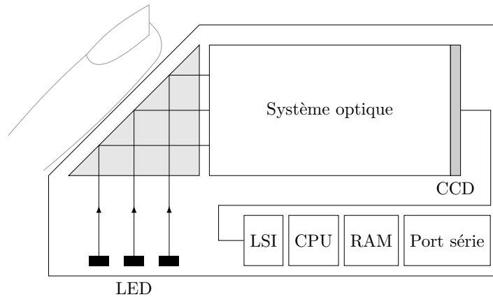
Figure 2 Principe d'un capteur optique d'empreinte digitale
