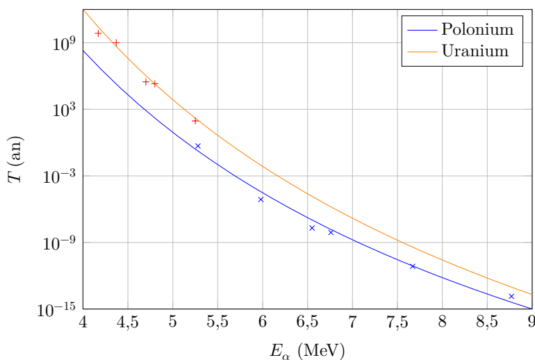
Figure 10 Demi-vie fonction de E_\alpha
