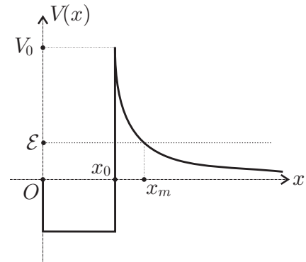
FIGURE 5 – Allure de l'énergie de potentielle
