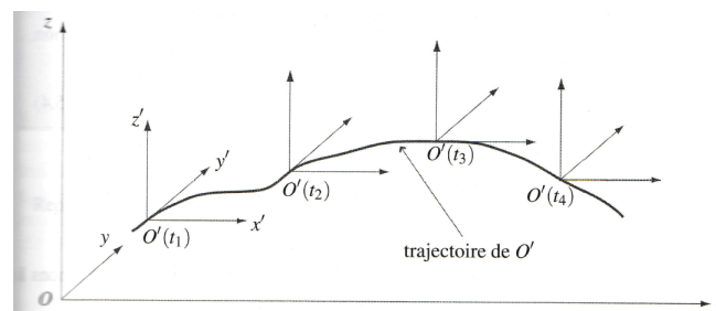
FIGURE 3 – Exemple de translation quelconque de \mathcal{R}' dans \mathcal{R} .
