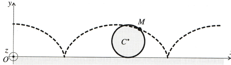
FIGURE 2 – Trajectoire de la valve d'une roue de vélo dans le référentiel terrestre.
