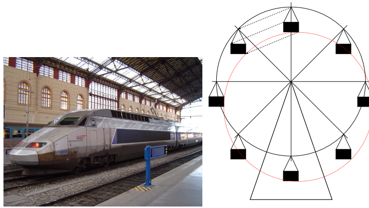
FIGURE 4 – Un référentiel lié au train est en translation rectiligne (non uniforme) par rapport au quai. Une nacelle d'une grande roue est en translation circulaire par rapport au sol, remarquer que la trajectoire de chaque point est un cercle de même rayon mais de centre différent.
