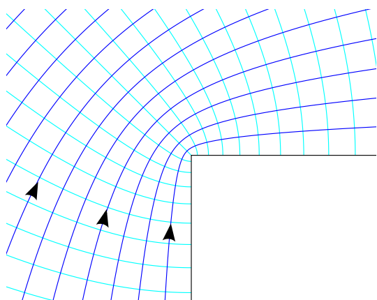
FIGURE 9 – Écoulement irrotationnel près d'une arête : lignes de courant (foncé), équipotentielles (clair).
