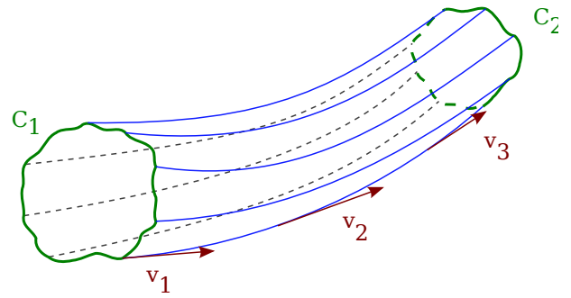
FIGURE 8 – Tube de courant appuyé sur C_1 .
