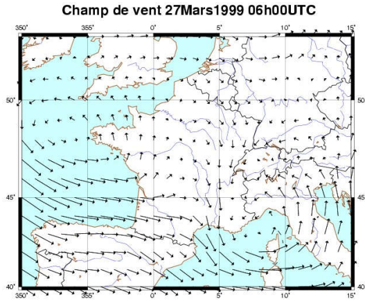
FIGURE 7 – Exemple de champ des vitesses.
