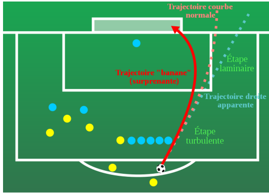
FIGURE 5 – Le 3 juin 1997, le Brésilien Roberto Carlos tire un coup franc à la trajectoire étonnamment courbée. Mais il fut expliqué ensuite par des chercheurs de Polytechnique (Guillaume Dupeux et al. 2010 New J. Phys. 12 093004).
