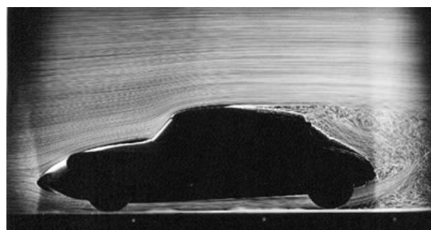
FIGURE 2 – L'écoulement est en général turbulent à l'arrière d'une voiture.
