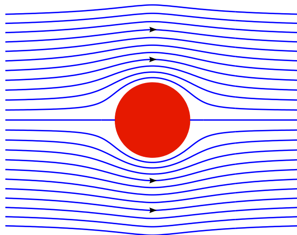
FIGURE 10 – Écoulement irrotationnel autour d'un cylindre.
