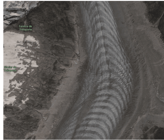
FIGURE 6 – Même les solides peuvent (lente-ment) s'écouler. Ici la « Mer de Glace » près du Mont Blanc. On reconnaît un champ des vitesses parabolique de type « Poiseuille ».
