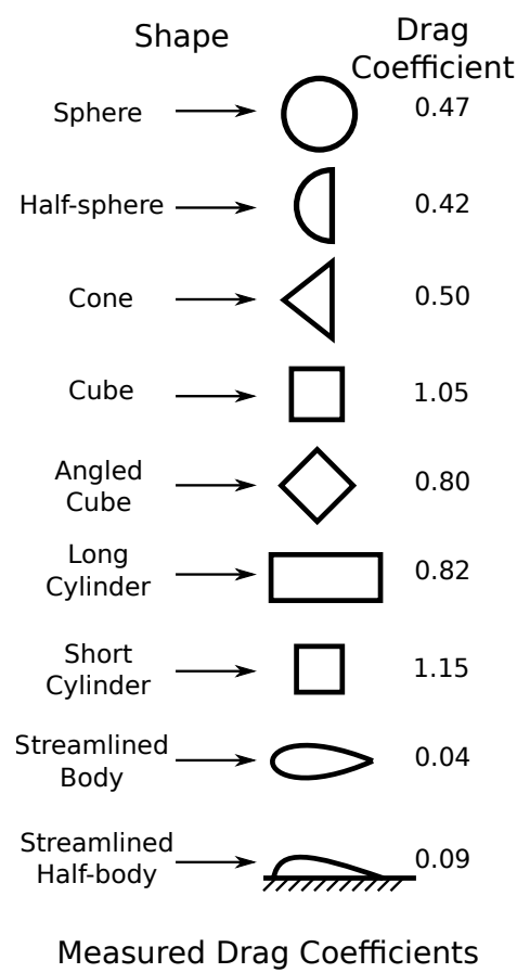
FIGURE 4 – Évolution du C_x en fonction de la forme du solide dans le régime en C_x dépend peu de v .
