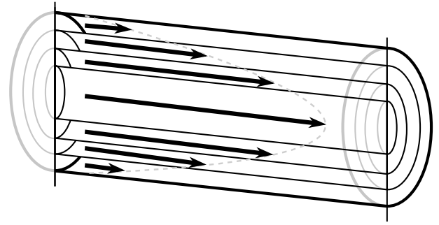
FIGURE 2 – Champ des vitesses d'un écoulement de Poiseuille cylindrique stationnaire. La vitesse est plus grande au centre.
