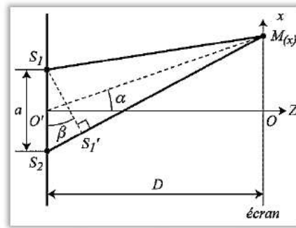
FIGURE 13 – Schéma du dispositif expérimental
