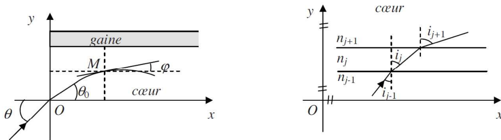
FIGURE 5 – Trajectoire du rayon lumineux dans une fibre à gradient d'indice.
