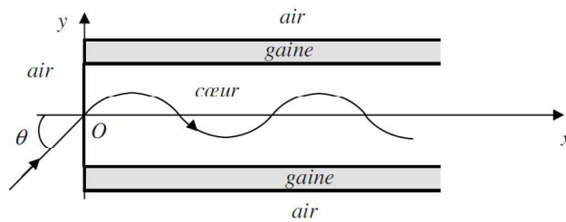
FIGURE 4 – Fibre optique à gradient d'indice.
