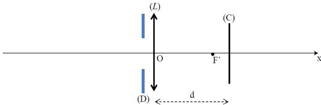
FIGURE 6 – Modélisation d'un appareil photographique.
