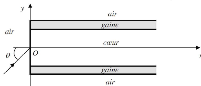
FIGURE 2 – Fibre optique à saut d'indice.
