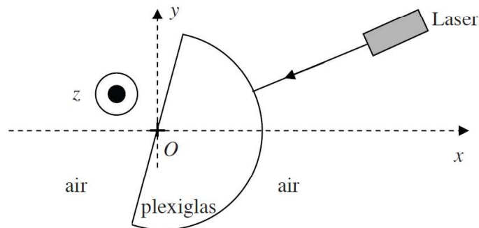
FIGURE 1 – Expérience avec un demi-cylindre de plexiglas.
