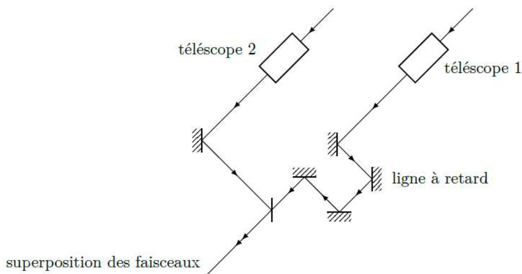
FIGURE 10 – Principe du VLTI.
