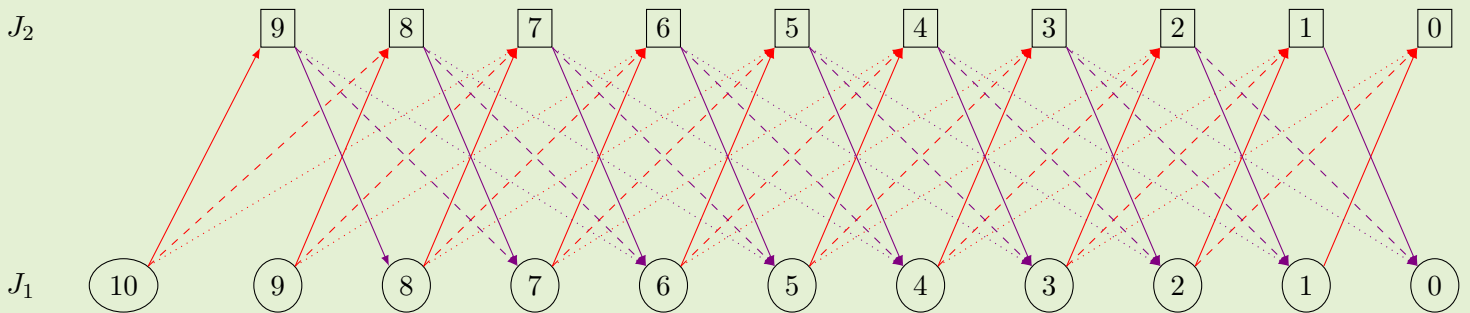
FIGURE 4 – Détermination de l'attracteur de J_1
