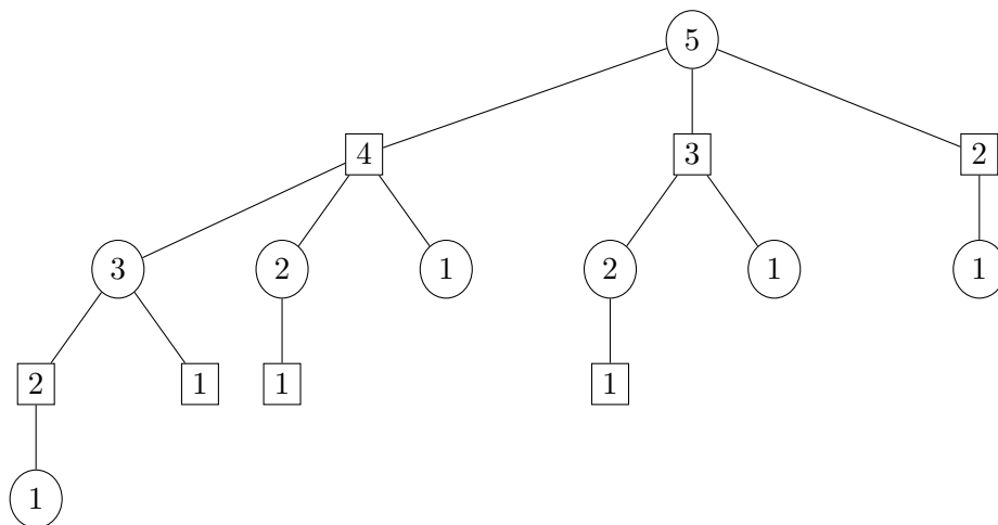
FIGURE 7 – Arbre de jeu.
