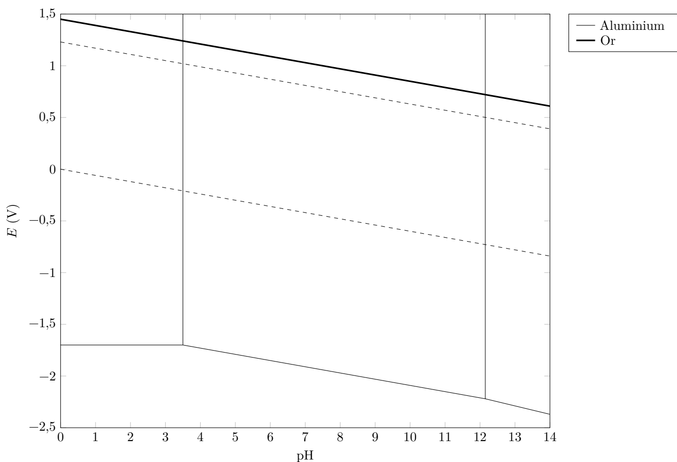
Figure A Diagrammes potentiel-pH de l'aluminium et de l'or ( T = 298 K)
