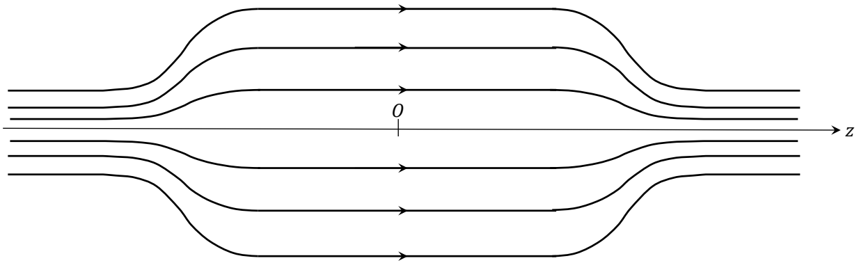
Figure 3 - Lignes de champ d'une bouteille magnétique
