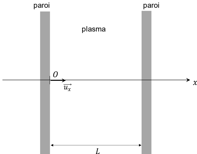
Figure 4 - Géométrie de l'enceinte contenant le plasma
