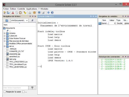
Figure 3 : Redémarrer Scilab
