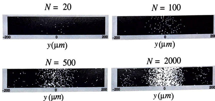
FIG. 6 – Distribution des impacts des neutrons sur l'écran
