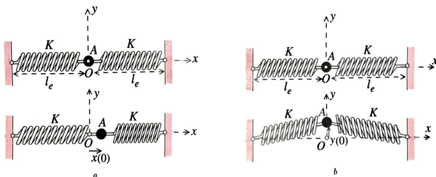
FIG. 1 – Oscillateur harmonique dans un plan horizontal Oxy (a) Déplacement longitudinal (b) Déplacement transversal
