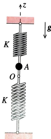
FIG. 2 - Oscillateur harmonique vertical
