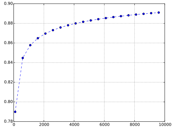
FIGURE 5 – Tracé de la suite (v_n)_n
