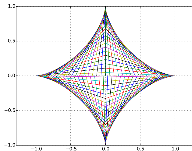
FIGURE 8 – Familles des segments d'extrémités (0, \cos(t)) , (\sin(t), 0)
