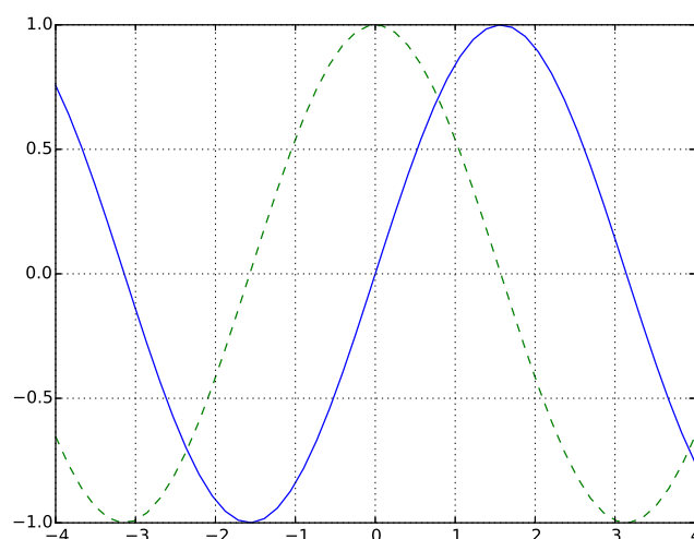
FIGURE 6 – Tracé de y = \sin(x) et y = \cos(x)
