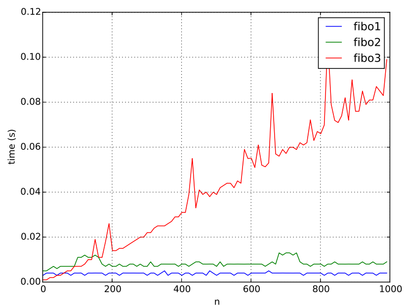
FIGURE 1 – Tracé des temps d'exécution du calcul de (u_n)_n
