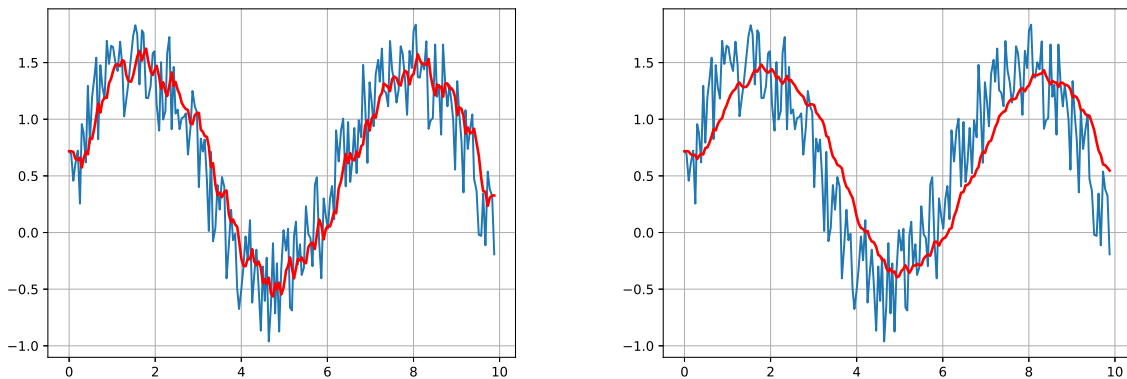
FIGURE 1 – Débruitage par filtre passe-bas RC pour différentes valeurs de \tau
