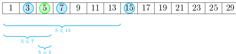
FIGURE 1 – Recherche dichotomique de 5 dans [1, 3, \dots, 29]
