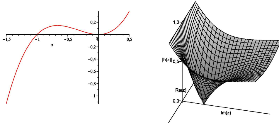
(a) Fonction g de l'exercice 1.24
