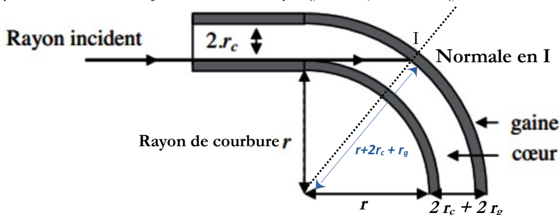
Figure 2 : Perte d'énergie dans une fibre optique courbée.
