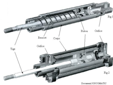
FIGURE 21 – Constitution d'un vérin.
