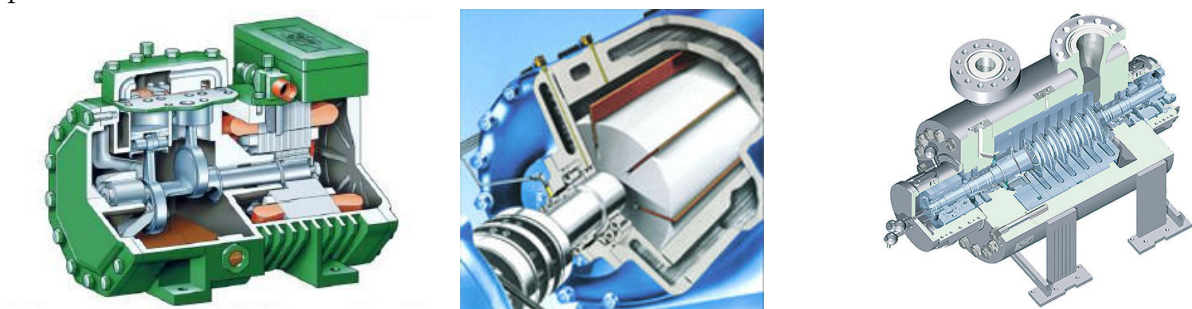
Compresseur alternatif
