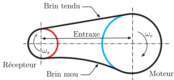
FIGURE 35 – Transmission par lien flexible.
