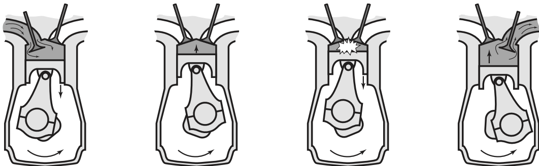
(a) Admission (b) Compression (c) Explosion, détente (d) Échappement
