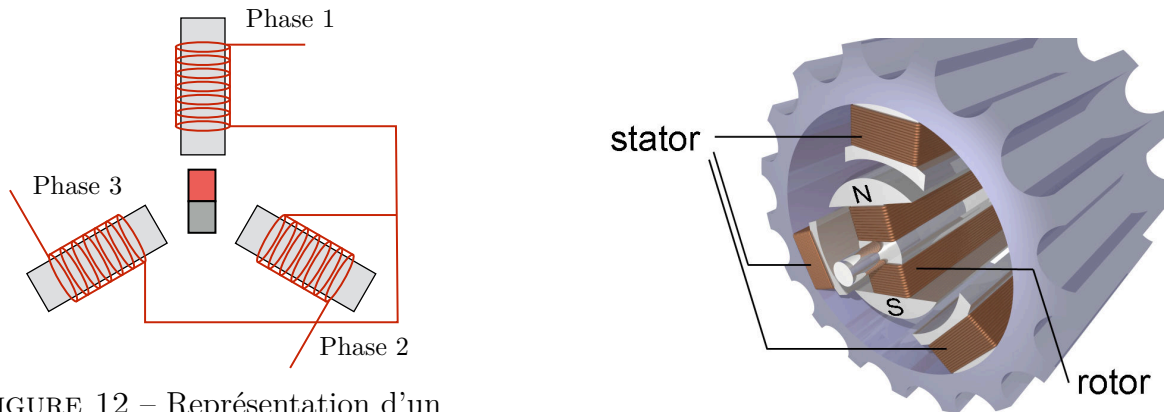
FIGURE 12 – Représentation d'un moteur synchrone.
