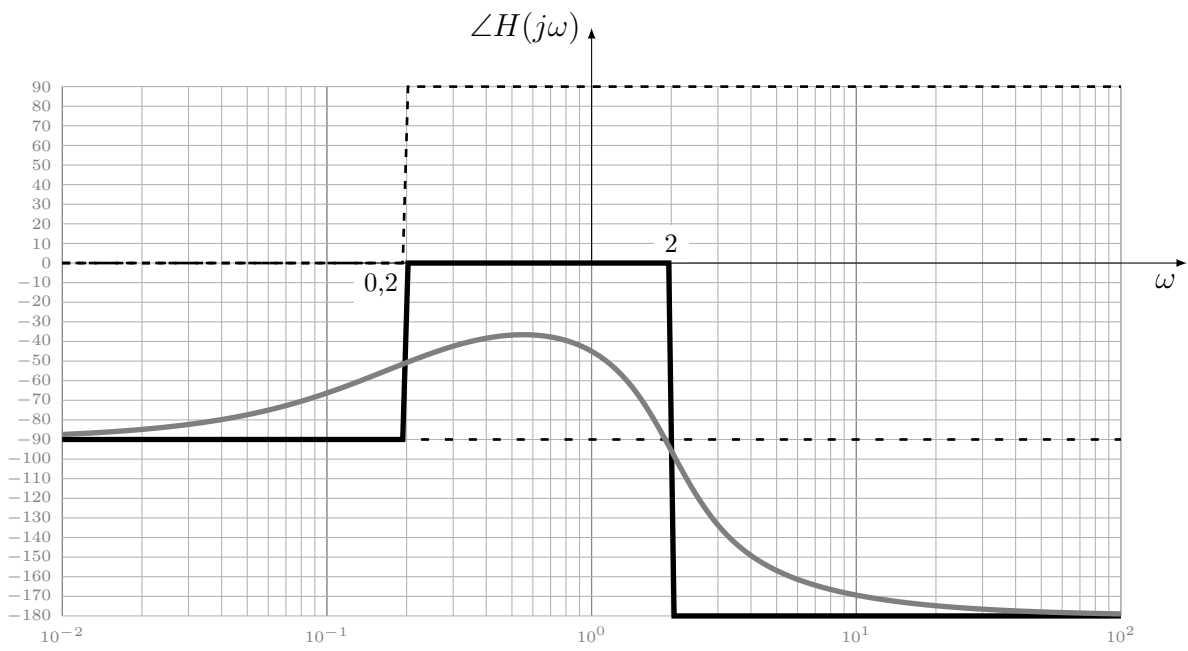
FIGURE 13 – Diagrammes de Bode de la fonction de transfert H(p) = \frac{5(1+2p)}{p(1+0,5p+0,25p^2)} .
